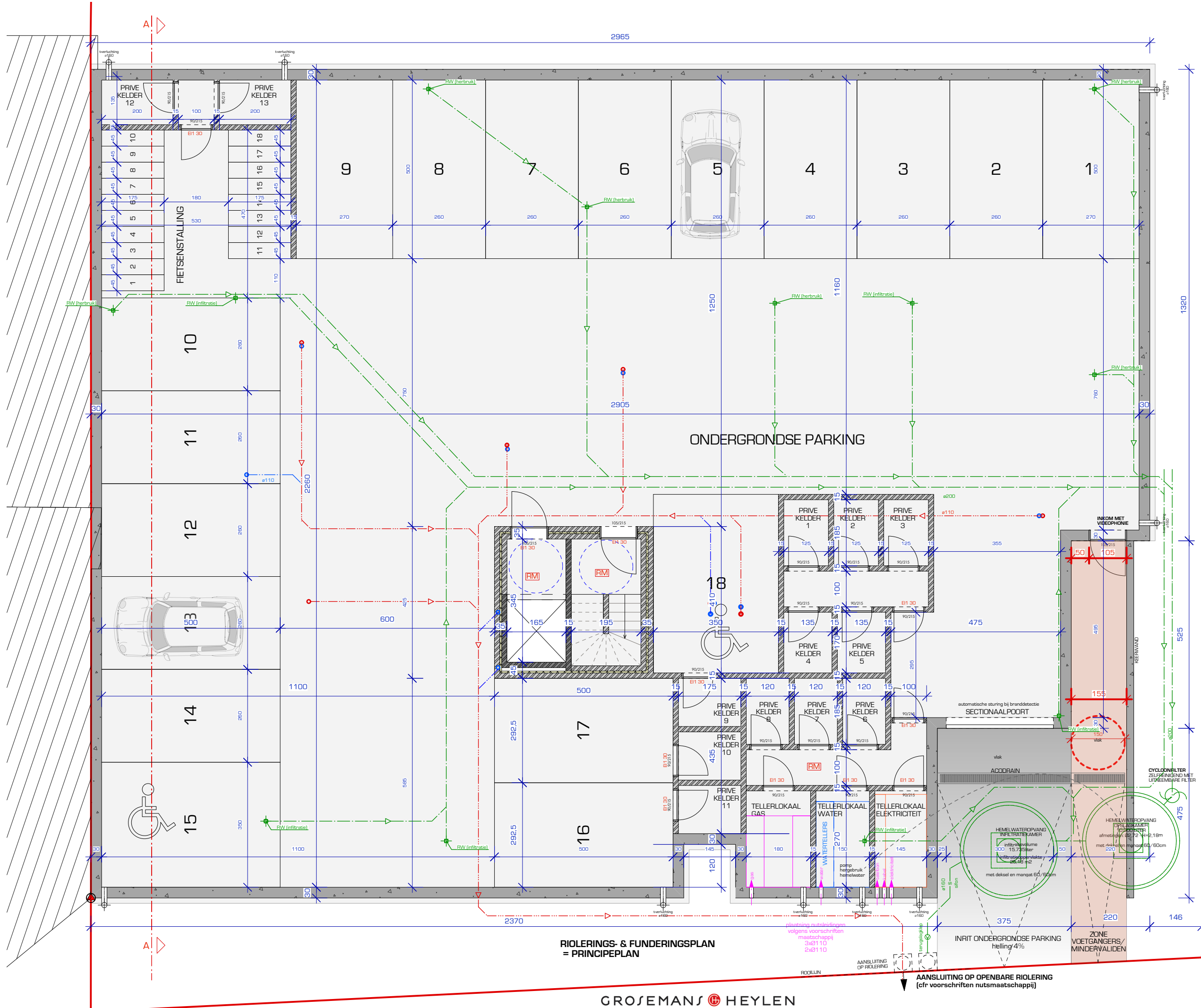
ONDERGRONDSE PARKING - RIOLERINGSPLAN Schaal 1 : 100
