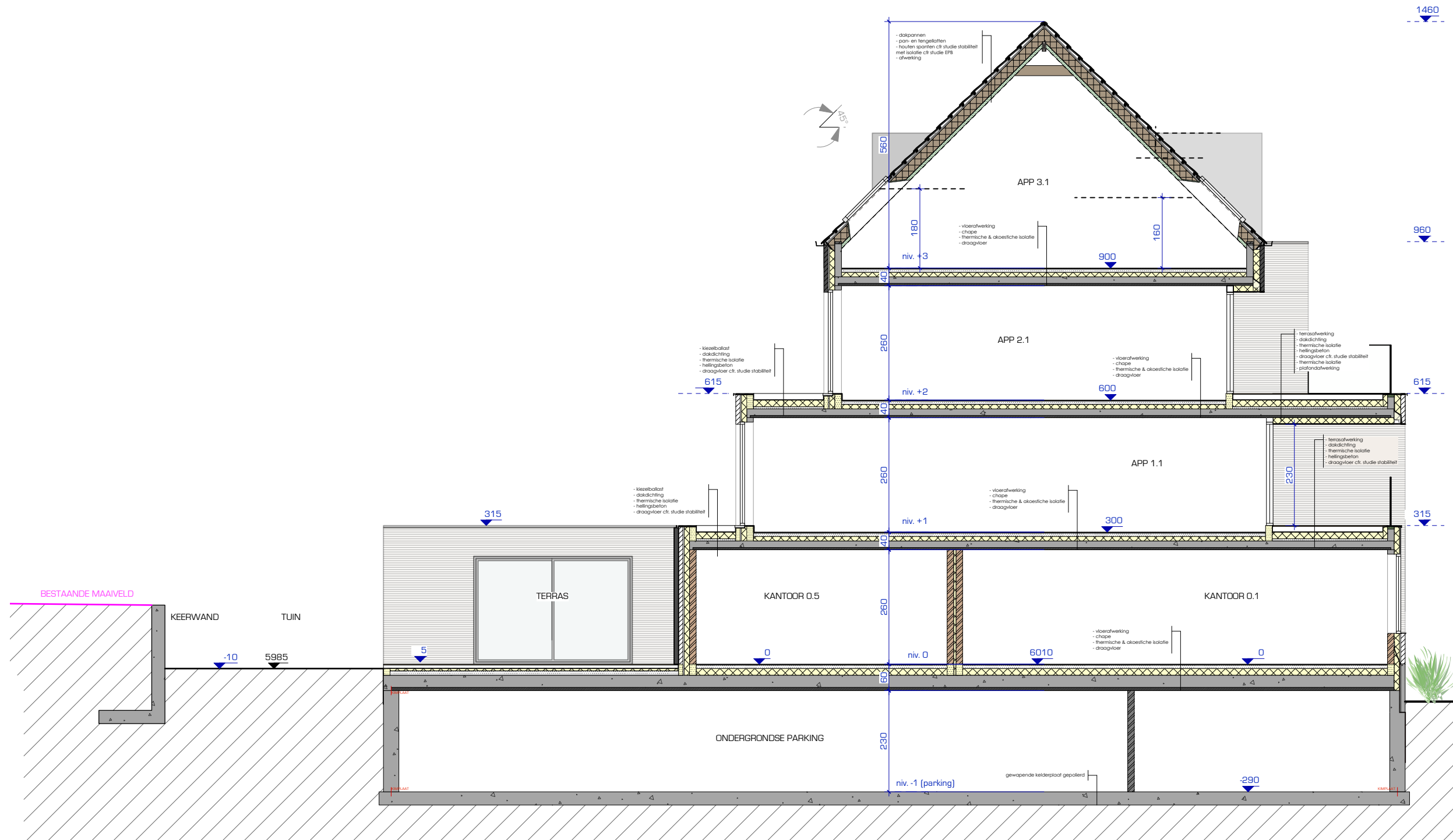
DOORSNEDE Schaal 1 : 100
